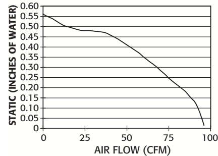
Fan Curve FV-08VQL3
