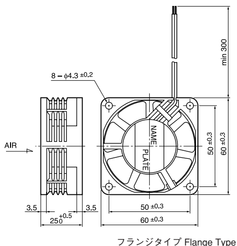
フランジタイプ Flange Type
