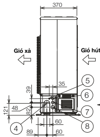
Hướng nhìn Z
