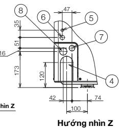
Hướng nhìn Z
