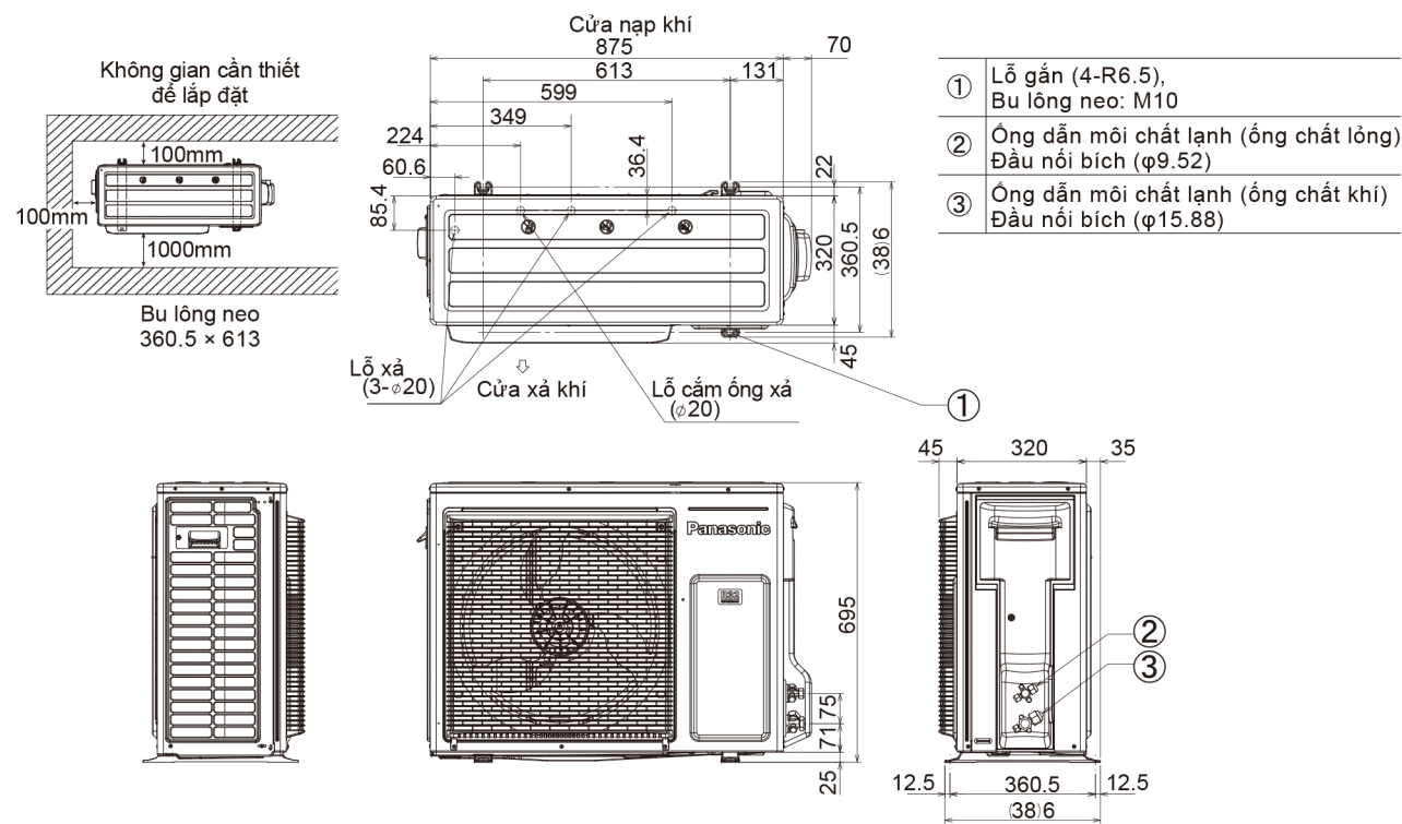
Kích thước (U-30PN1H5) 1-pha (U-30PN1H8 / U-36PN1H8) 3-pha
