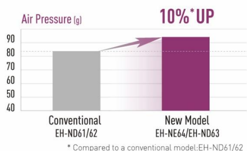
气压性能
