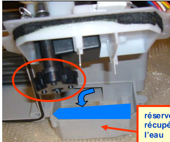
Pompe de vidange vue de dessous
