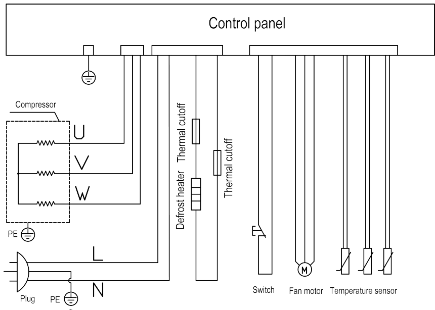
电路原理图
