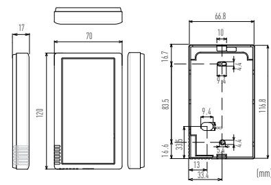
REMOTE SENSOR (CZ-CSRC3)
