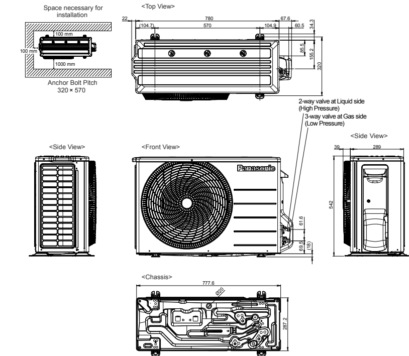
Dimensions (2.5kW – 2.6kW) CU-Z25UBRA
