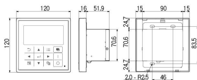
系統控制器(CZ-64ESMC3)
