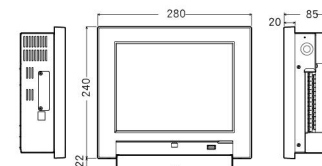
智慧型控制器(CZ-256ESMC3)
