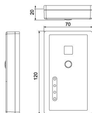
系統控制器(CZ-64ESMC3)
