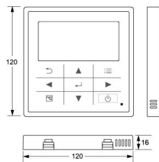
高規格有線遙控器(CZ-RTC5A)
