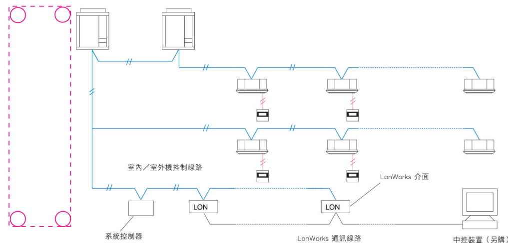
系統範例圖LonWorks介面
