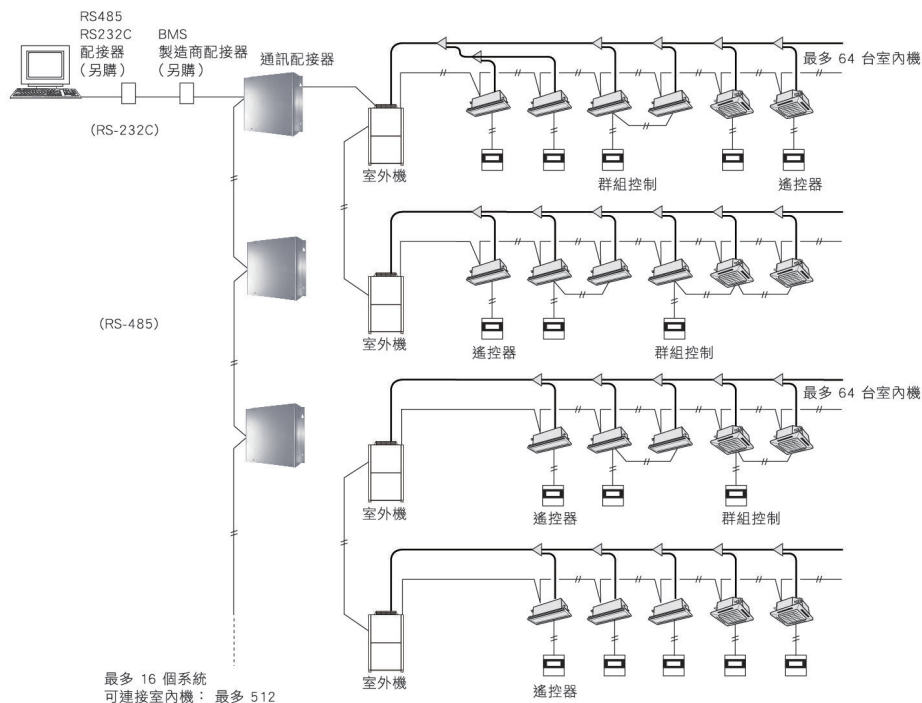
第三方BMS與CZ-CFUNC2連接範例圖（詳細資訊請洽授權經銷商）
