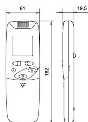
簡易式遙控器(CZ-RE2C2)
