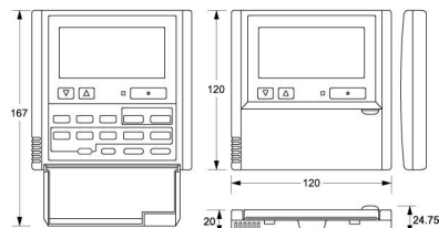
有線遙控器(CZ-RTC4)
