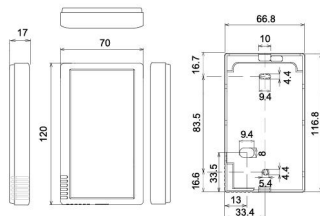
遠端感應器(CZ-CSRC3)
