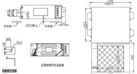
接線配置圖*1 FY-E15DZ1AW控制器另購
