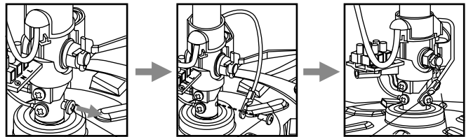
Tighten the Safety Wire Screw 鎖緊保險線螺絲 Vặn chặt vít dây an toàn
