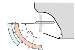
Heating: F1 to F5 Cooling: F1 to F3
