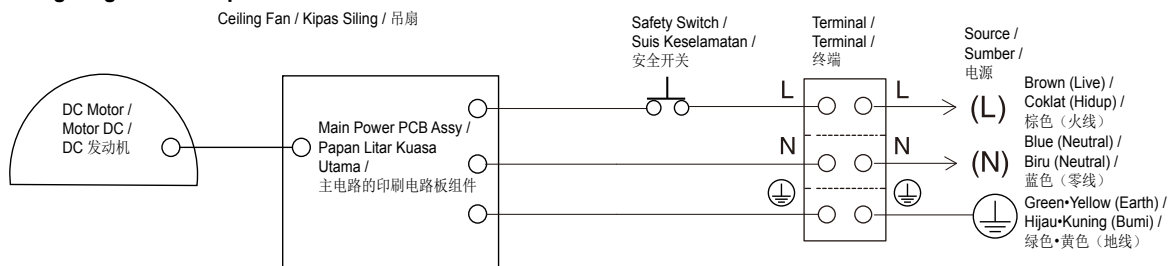
Wiring diagram / Litar pendawaian / 电线图
