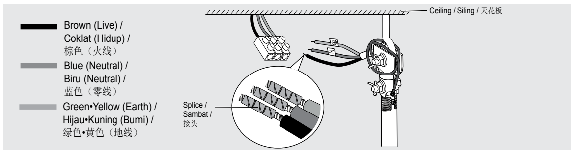
Wiring diagram / Litar pendawaian / 电线图
