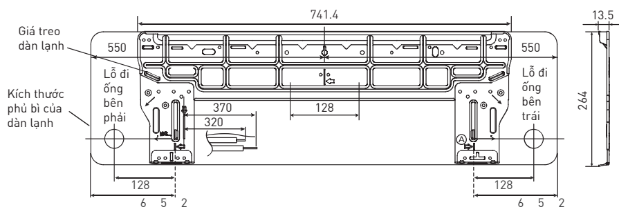
Vị trí tương đối giữa dàn lạnh và giá treo dàn lạnh <Mặt trước>
