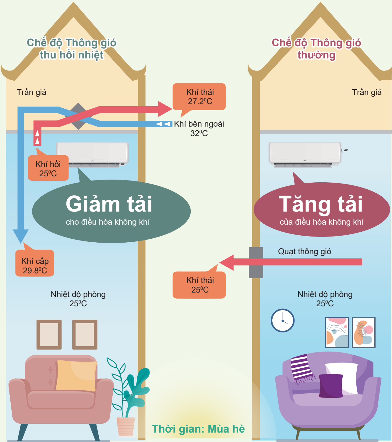
Tận dụng nhiệt độ thấp của khí hồi bên trong ngôi nhà để làm mát khí bên ngoài nhờ thiết bị trao đổi nhiệt
