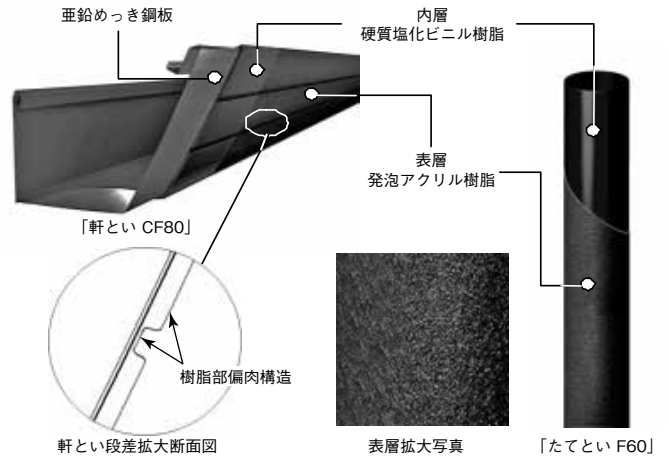
図1 住宅用雨とい「フォルティガ」の構成
